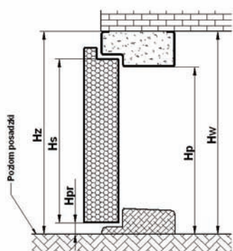
Ościeżnica drzwi, próg
