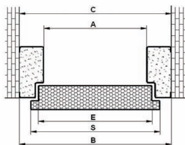
Ościeznica drzwi
