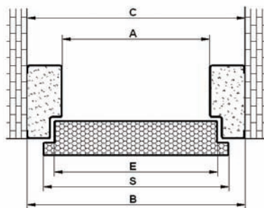
Ościeżnica drzwi
