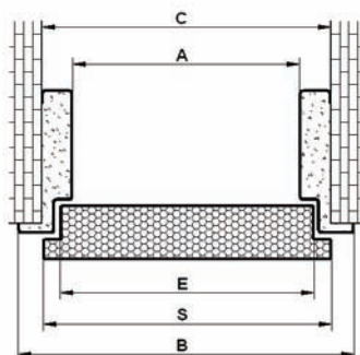
Ościeznica drzwi
