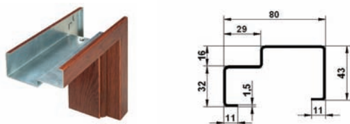
OŚCIEŻNICA ASYMETRYCZNA BEZ USZCZELKI FB (do drzwi TT i GTT)
