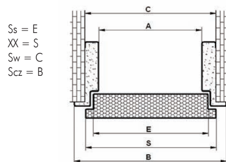
Ościeżnica drzwi
