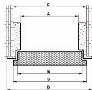
Ościeżnica drzwi
