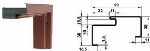
OŚCIEŻNICA ASYMETRYCZNA Z USZCZELKĄ FA (do drzwi TT, GTT)
